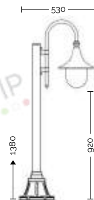
1944A/1L 1944A/2L B3 - P20
