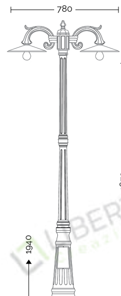
1594/1L 1594/2L 1594/3L B28-P05
