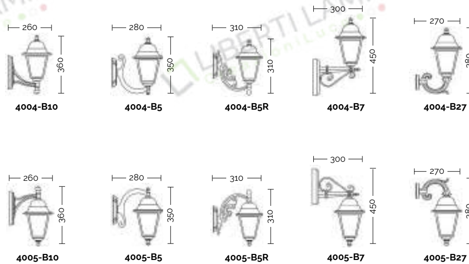
(*) 4000 LANTERNA A PARETE (diffusore: policarbonato) (diffuser: polycarbonate)
